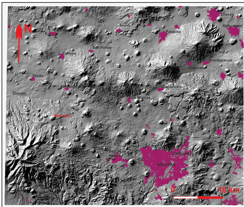
Figura 5. Modelo digital de sombras de la Región Volcánica del Parícutin (RVP). Imagen generada a partir de la base de datos de relieve del INEGI, de las hojas Uruapan (E13B39), Paracho (E13B29), Cherán (E14A21) y Taretan (E14A31), escala 1:50 000.
