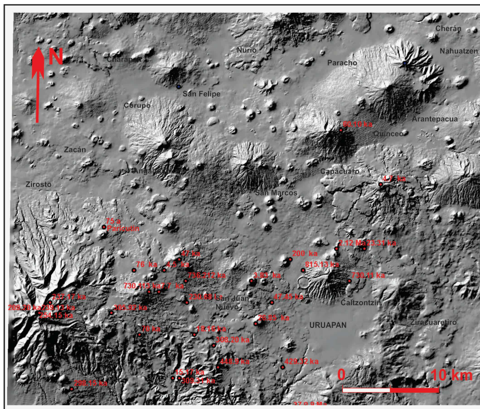
Figura 7. Modelo digital de elevaciones de la Región Volcánica del Parícutin y la proyección de los diferentes fechamientos isotópicos. Los datos fueron compilados por diversos autores y se presentan en material suplementario 3 (RVP_supl.3).
