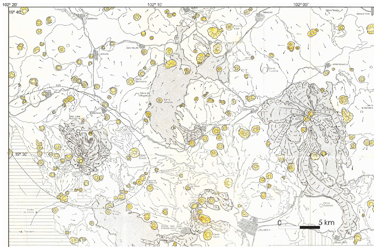
Figura 4 Mapa vulcanológico de la Región Volcánica del Parícutin (modificado de Demant, 1981). Notar que los dibujos interpretados de los conos volcánicos han sido resaltados con amarillo. Notar también el límite elipsoidal de influencia de las cenizas volcánicas del Parícutin (Segerstrom, 1950).
