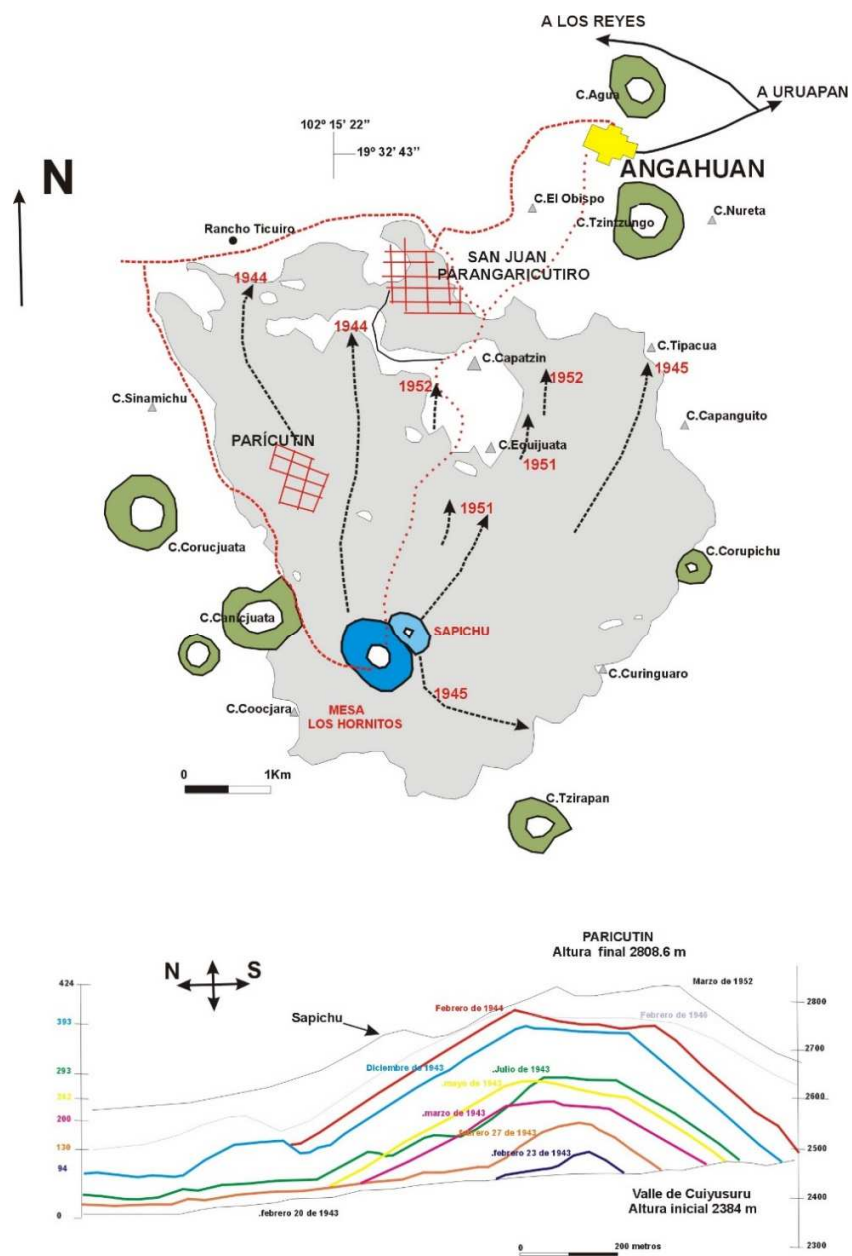
Figura 3. Principales derrames de lava históricos del Parícutin y perfil que muestra las diferentes etapas de crecimiento del Volcán Parícutin, después de Foshag y Reyna (1956). Figura modificada de Corona-Chávez (2002).
